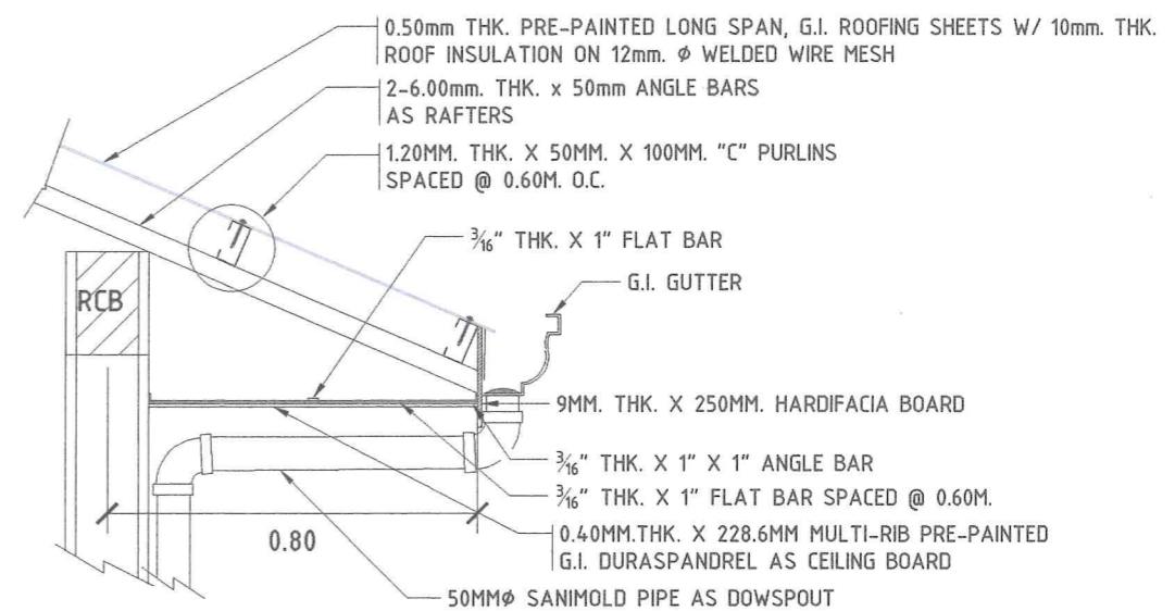
EAVES DETAILS SCALE : 1 : 20 MTS.
