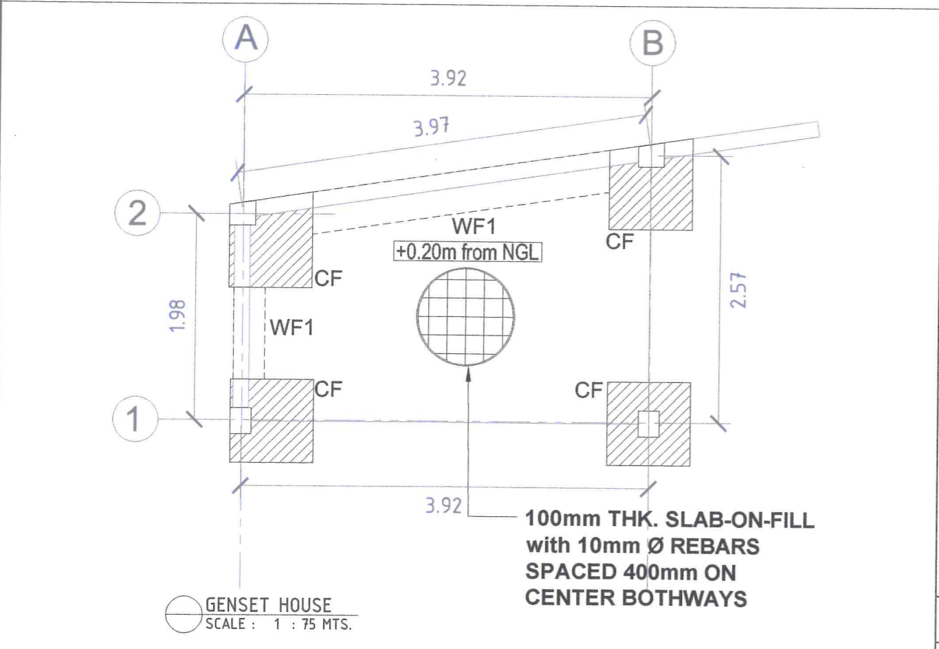
FOUNDATION PLAN SCALE : 1 : 75 MTS.
